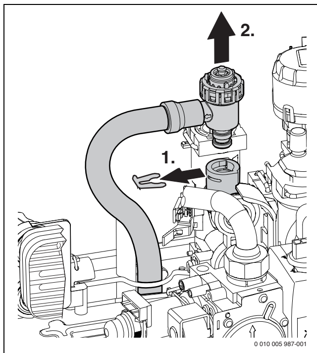
Сурет 34 Сақтандыру клапанын шешіңіз (жылыту контуры)
