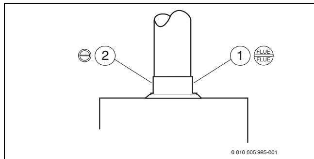
Сурет 32 Пайдаланылған газдар мен жанатын ауаны өлшеуге арналған штуцер
