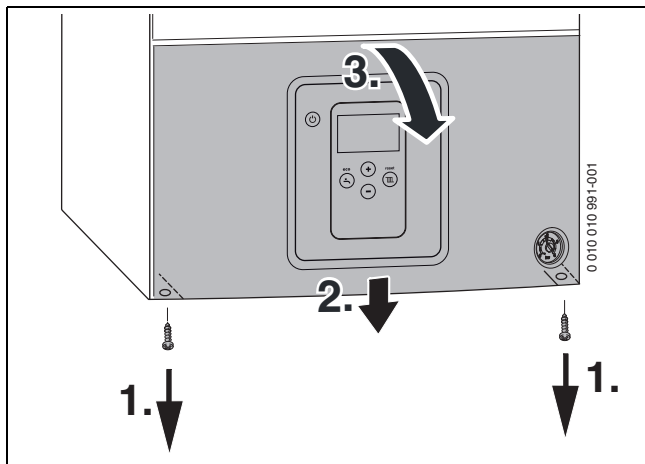
Сурет 15 Басқару блогын төмен түсіріңіз
