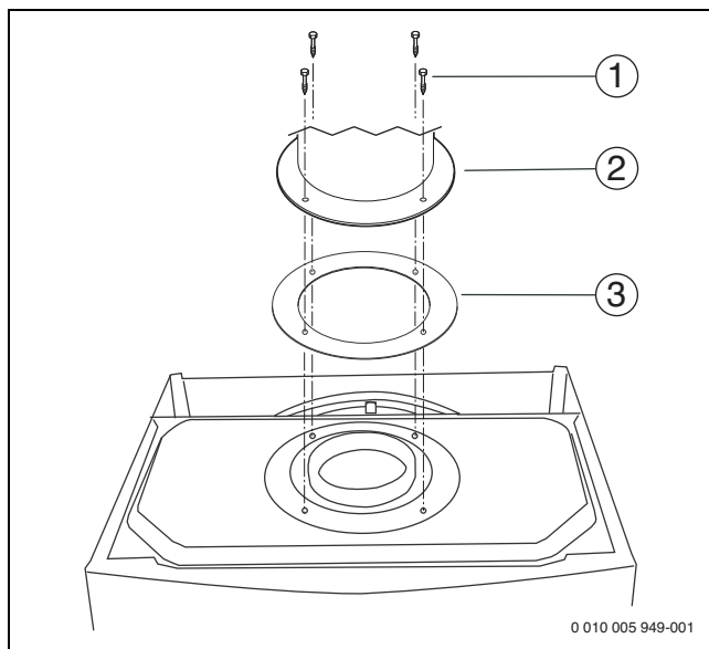
Сурет 16 Пайдаланылған газға арналған керек-жарақтарды бекіту
