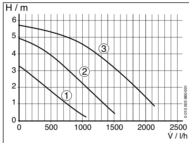
Сурет 28 Жылыту жүйесі сорғысының графикалық сипаттамасы (құрал қуаты < 35 кВт)
