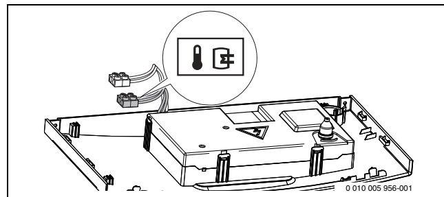
Сурет 23 Ресивердің температура датчигін қосыңыз
