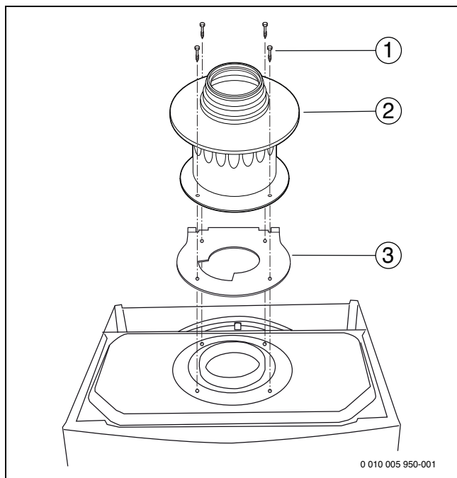
Сурет 17 Пайдаланылған газдарға B_{22} арналған құбыр желісі және аспап қуаттылығы < 35 кВт болғанда: пайдаланылған газдарды шығару жүйесі үшін адаптер және дроссельдік бөгет орнатыңыз
