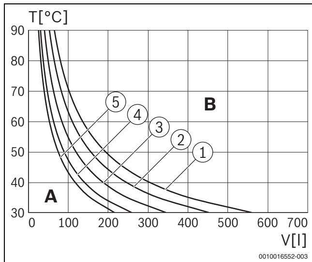
Сурет 11 Кеңейткіш ыдысының сипаттамасы 6 л. (Құрылғы қуаты <35 кВт)
