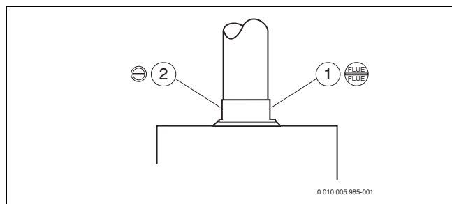
Рис. 32 Штуцер для измерения дымовых газов и штуцер для измерения воздуха для горения
