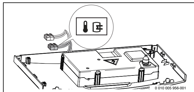
Рис. 23 Подключение датчика температуры бака-водонагревателя
