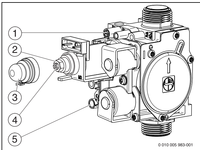
Рис. 31 Газовая арматура
