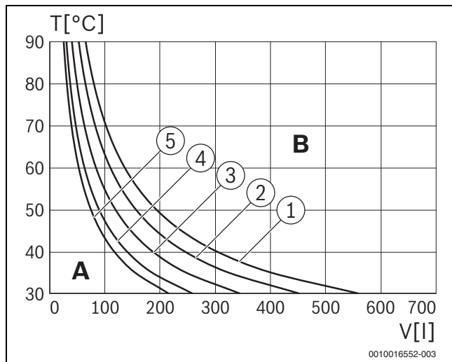
Рис. 11 Характеристики расширительного бака 6 л (мощность котла < 35 кВт)
