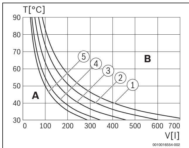
Рис. 12 Характеристики расширительного бака 8 л (мощность котла = 35 кВт)
