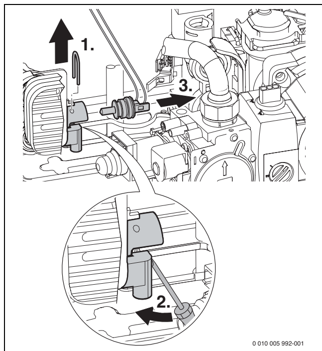
Рис. 39 Демонтаж датчика температуры горячей воды
