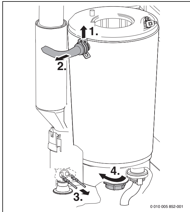
Рис. 64 Отсоедините трубу подающей линии и провода
