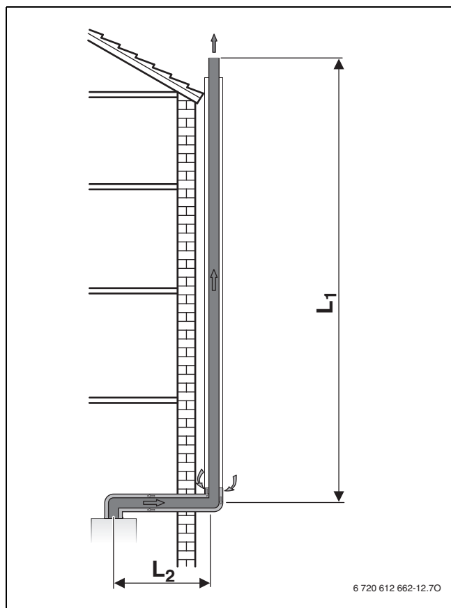
Рис. 15 Дымовая труба по фасаду по C_{53(x)}
