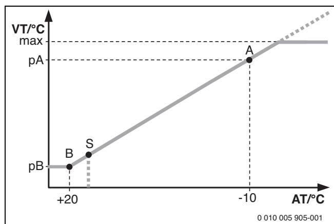
Рис. 67 Отопительная кривая
