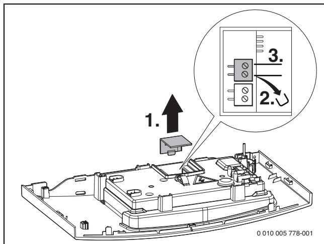
Рис. 27 Подключение регулятора
