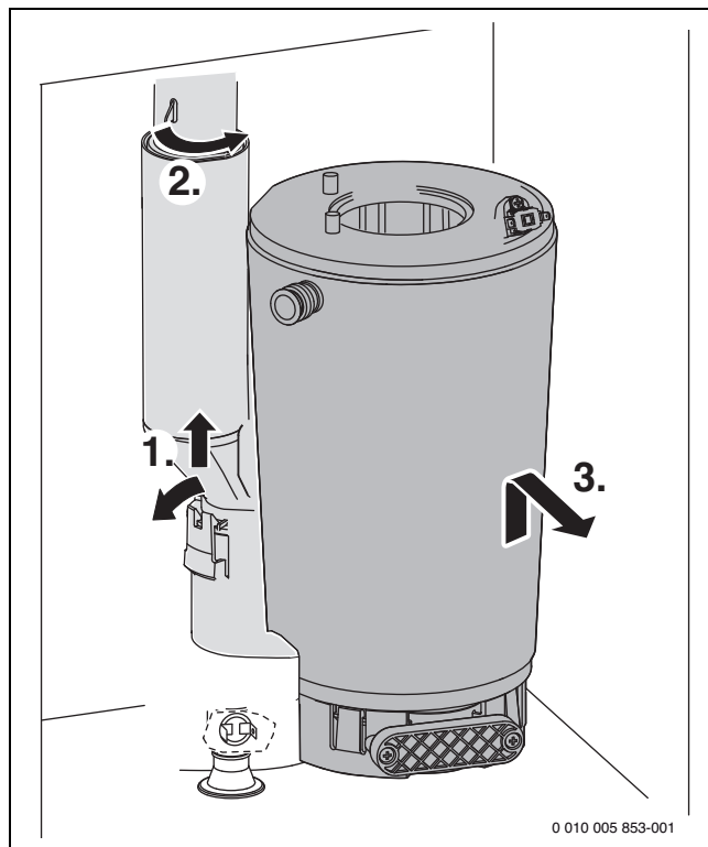
Рис. 65 Демонтаж теплообменника
