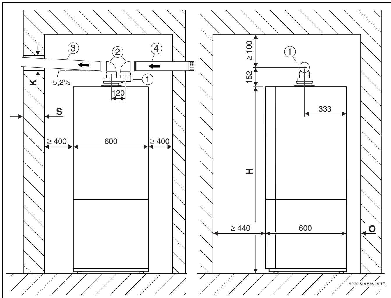
Рис 11 Ø 80/80 mm
