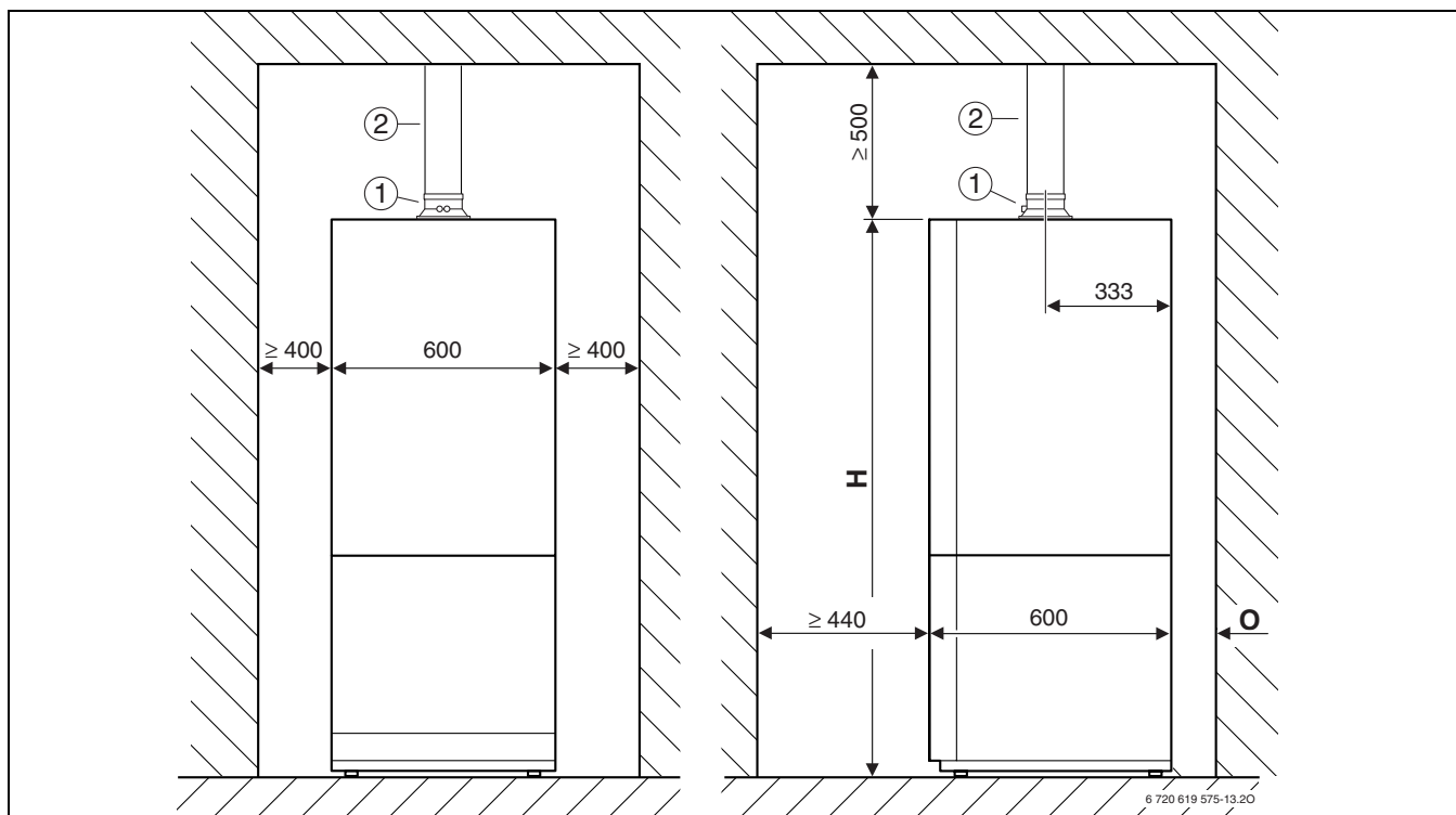
Рис 9 Ø 60/100 мм, плоская крыша
