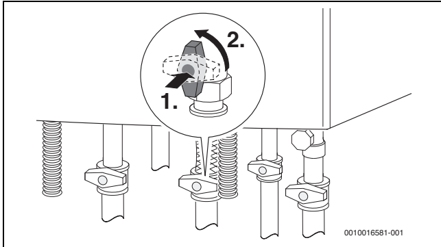
Рис. 5 Открытие газового крана
