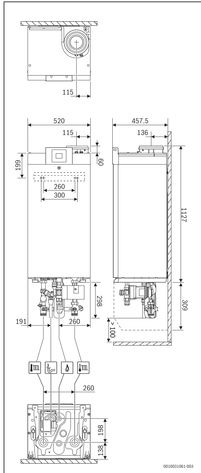
Сурет 3 Қабырғадағы өлшемдер [мм]
