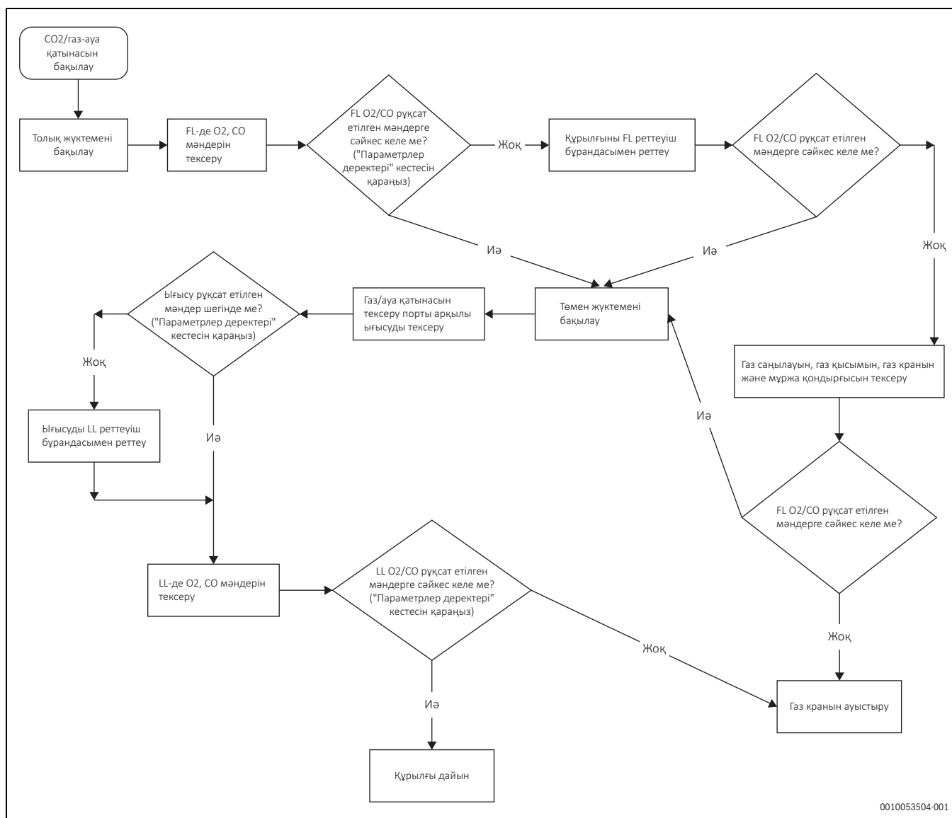
Сурет 35 Түзету нұсқауларының технологиялық сызбасы
