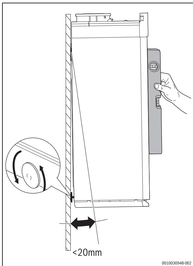
Сурет 12 Жылытқыш қазанды қабырғада туралау
