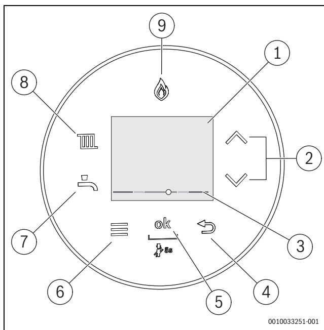
Сурет 37 Басқару панелі
