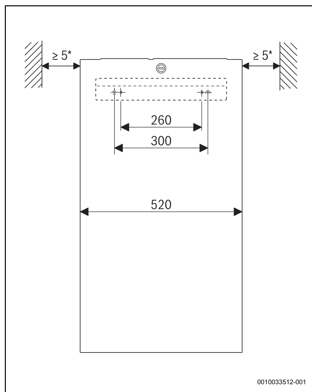
Сурет 5 Алдыңғы көрініс [мм]
