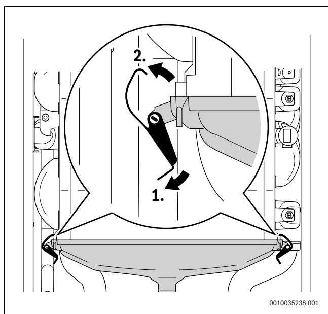
Сурет 46 Конденсатты жинау науасының ысырмалы бекіткіштерін ашыңыз.
