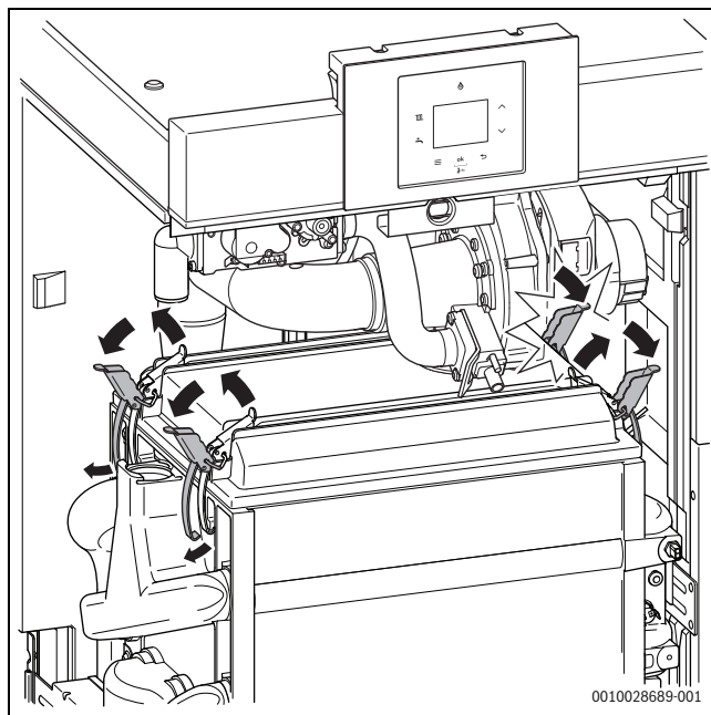
Сурет 40 Ысырмалы бекіткіштерді ашыңыз
