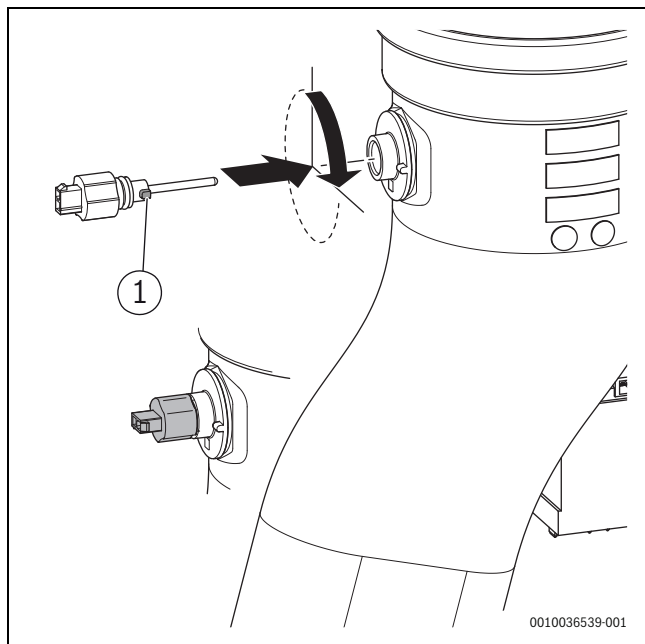
Сурет 49 Түтін газының температура датчигін ауыстыру
