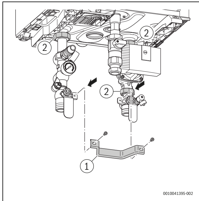
Сурет 15 Кронштейндерді монтаждаңыз
