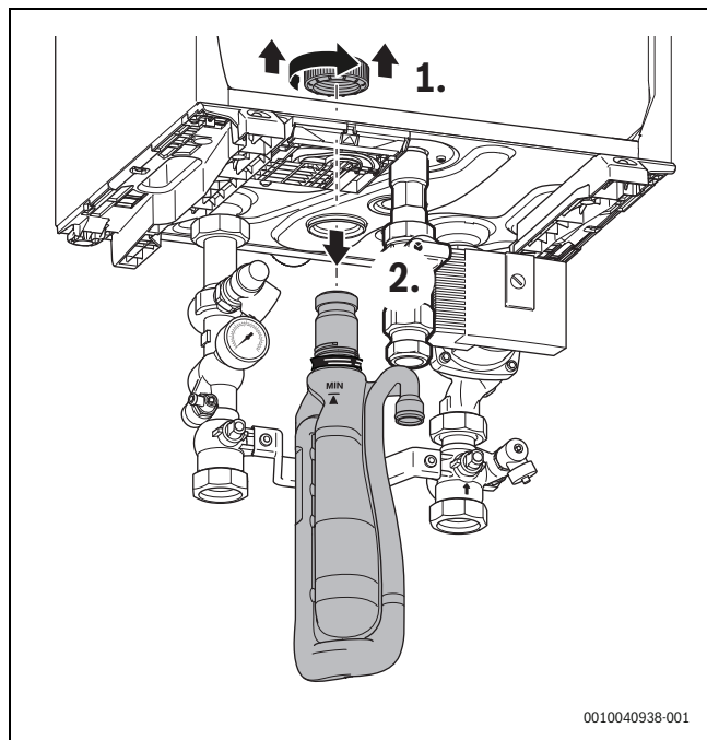
Сурет 45 Жылытқыш қазан сифонын алыңыз
