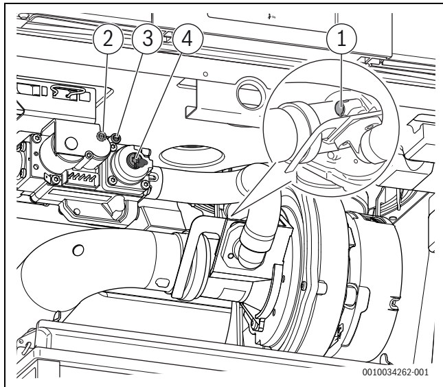
Сурет 32 Тексеру порттары мен реттеуіш бұрандаларға шолу \leq 70 кВт
