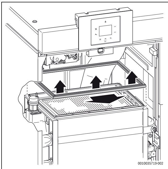
Сурет 42 Жанарғы тығыздағышын алу
