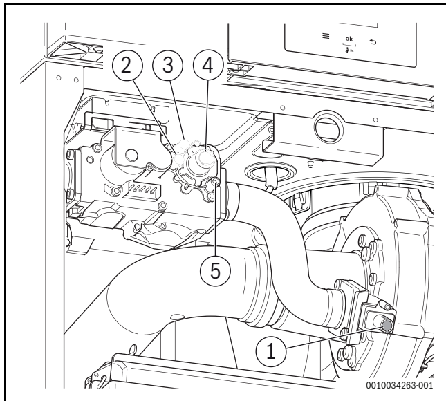
Сурет 33 Тексеру порттары мен реттеуіш бұрандаларға шолу \geq 85 кВт
