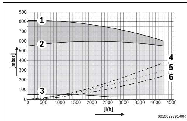
Сурет 53 Сорғының қалдық жылуы 85kW ≤ 100kW
