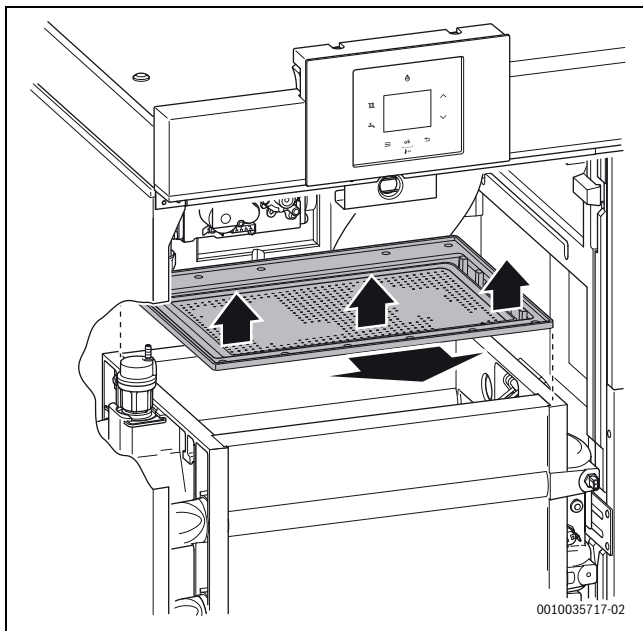
Сурет 43 Жанарғыны алу
