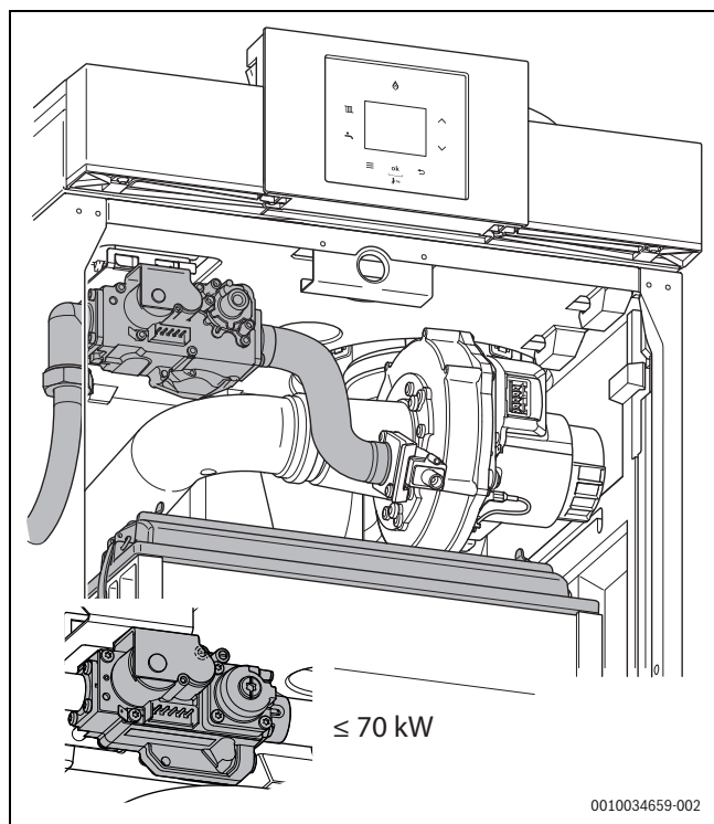
Сурет 36 Газ жолын тексеру
