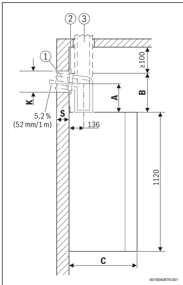
Сурет 4 Жанынан қарағандағы көрініс [мм]
