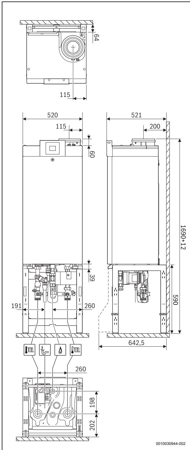
Сурет 2 Негізгі жақтаудағы өлшемдер [мм]
