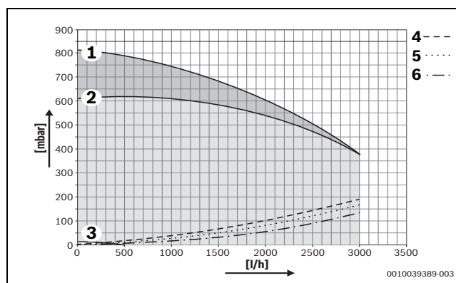
Сурет 52 Сорғының қалдық жылуы 50kW &lt; 85kW
