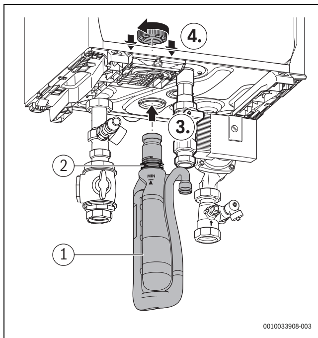
Сурет 16 Жылытқыш қазан сифонын монтаждау
