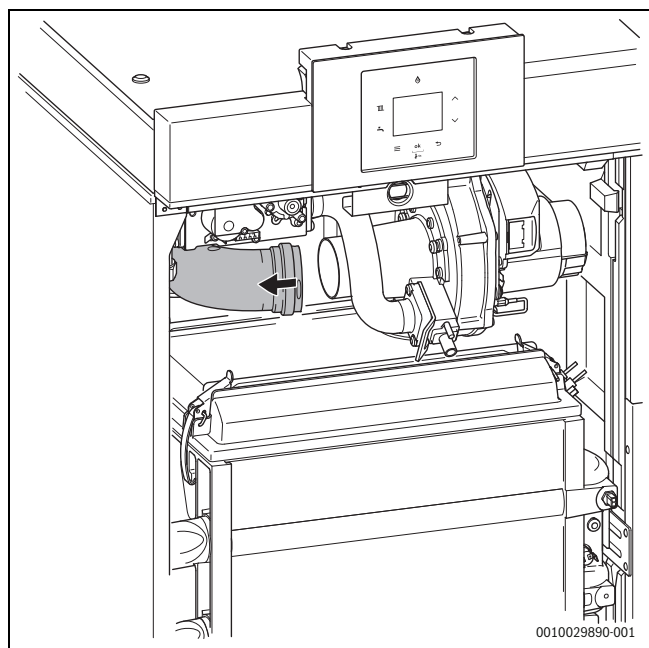
Сурет 39 Ауа қабылдау түтігін алу
