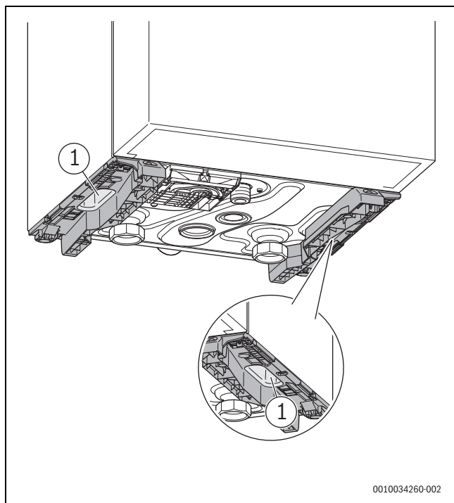
Сурет 7 Тұтқаларға арналған ойықтардың орналасуы
