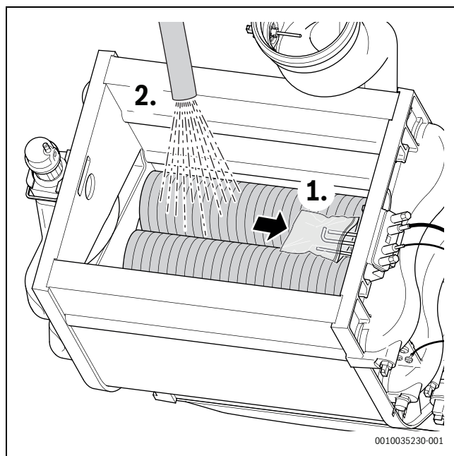
Сурет 44 Жылу алмастырғышты тазалау
