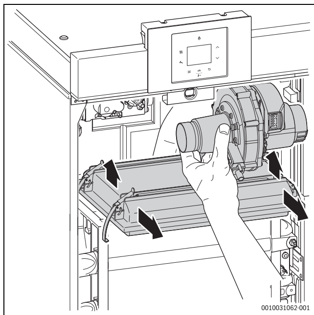
Сурет 41 Газ-ауа блогын жанарғы қаптамасымен бірге алыңыз.
