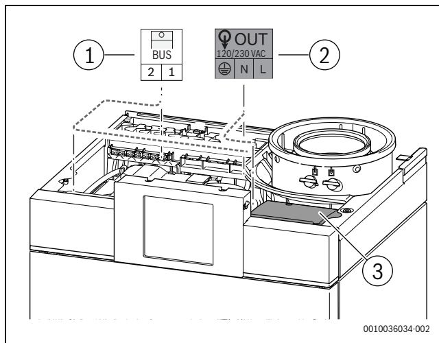
Сурет 30 Функционалдық модульді монтаждау
