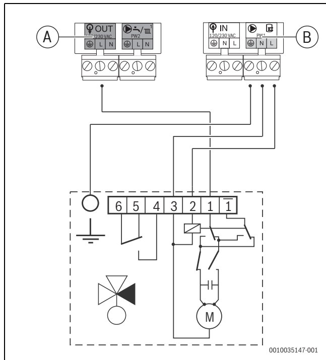
Сурет 29 230 В 3 жүрісті клапанды қосу схемасы
