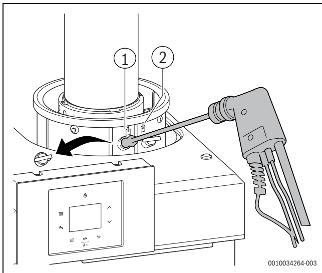
Сурет 34 Түтін мұржасындағы ашаны алыңыз
