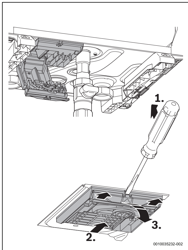
Сурет 25 Сорғының терминал блогын ашу
