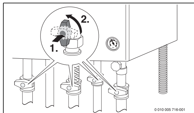
Рис. 2 Откройте сервисные краны
