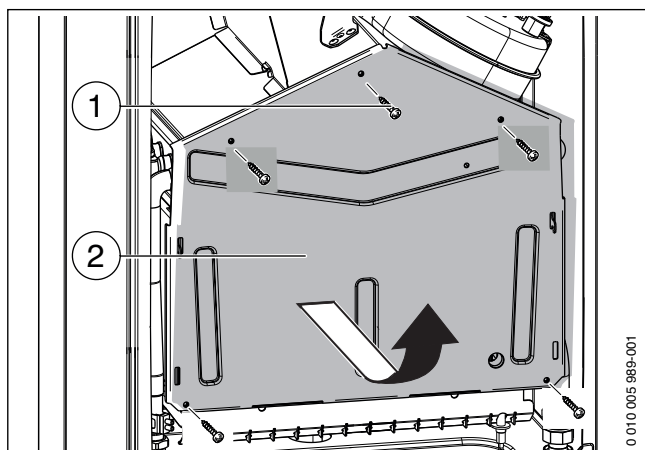
Рис. 31 Открытие горелки
