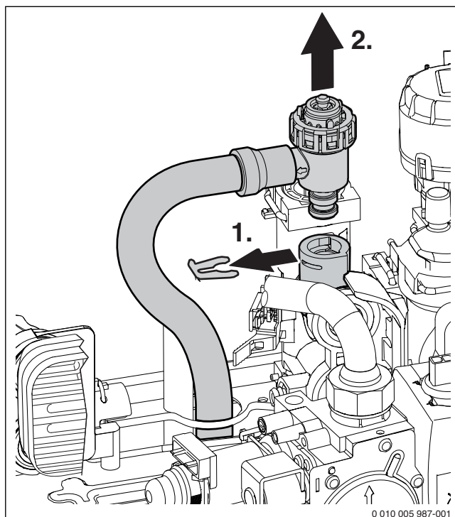
Рис. 29 Демонтаж предохранительного клапана (отопительного контура)
