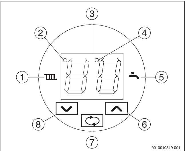
Рис. 3 Панель управления
