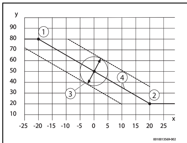
Рис. 4 Отопительная кривая зависимости температуры подающей линии от наружной температуры
