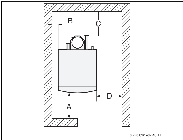
Сурет 8 Ұсынылатын қабырғамен арадағы қашықтық [мм] (жақшаға алынған минималды қашықтық)
