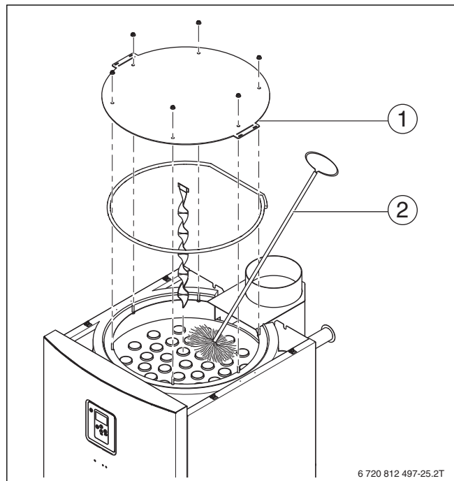
Сурет 36 Жағылатын газдардың жолдарын тазарту
