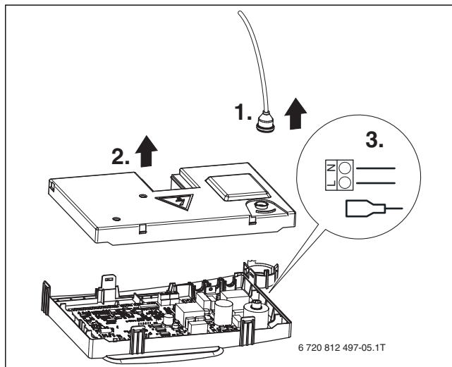
Сурет 20 Ыстық су сорғысын қосу
