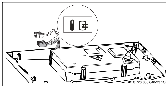
Сурет 16 Температура датчигін қосу
