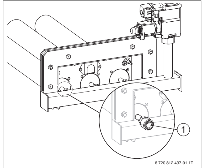
Сурет 24 Негізгі газ форсункаларын бақылау
